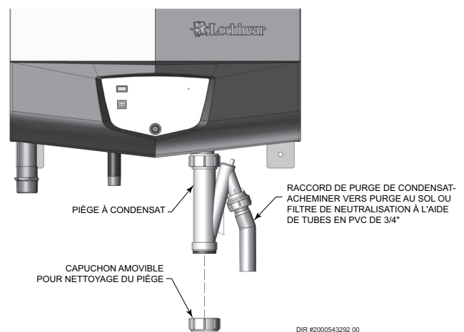
Figure 2-2 Rejet du condensat
